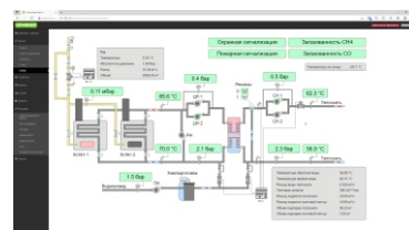
Интерактивная мнемосхема
