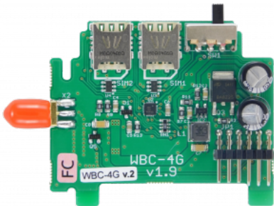
Обратная сторона модуля WBC-4G v.2 для WB6 и WB7
